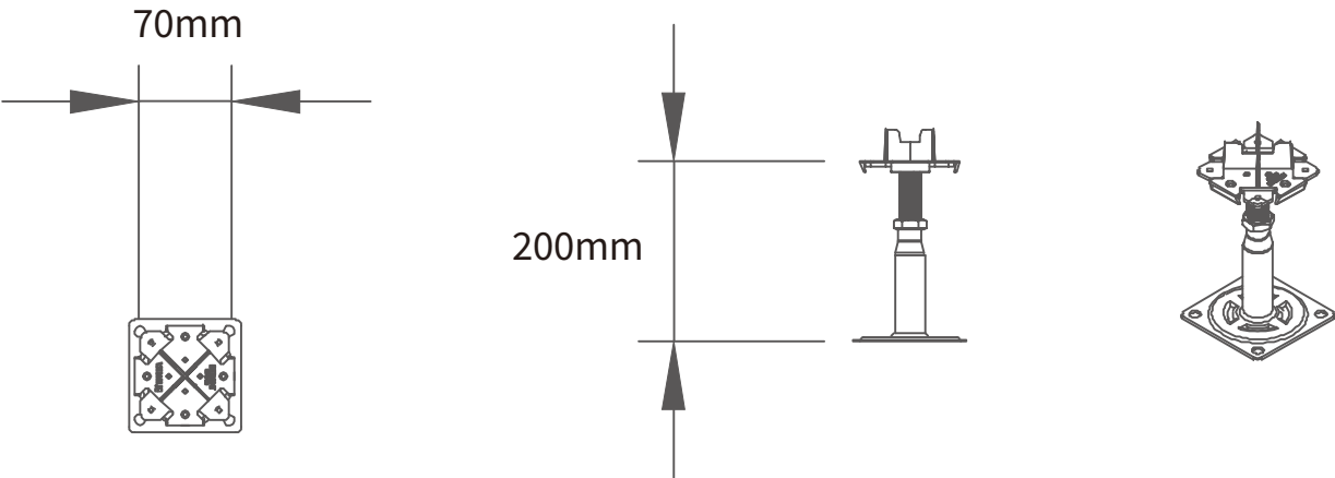
支架尺寸
